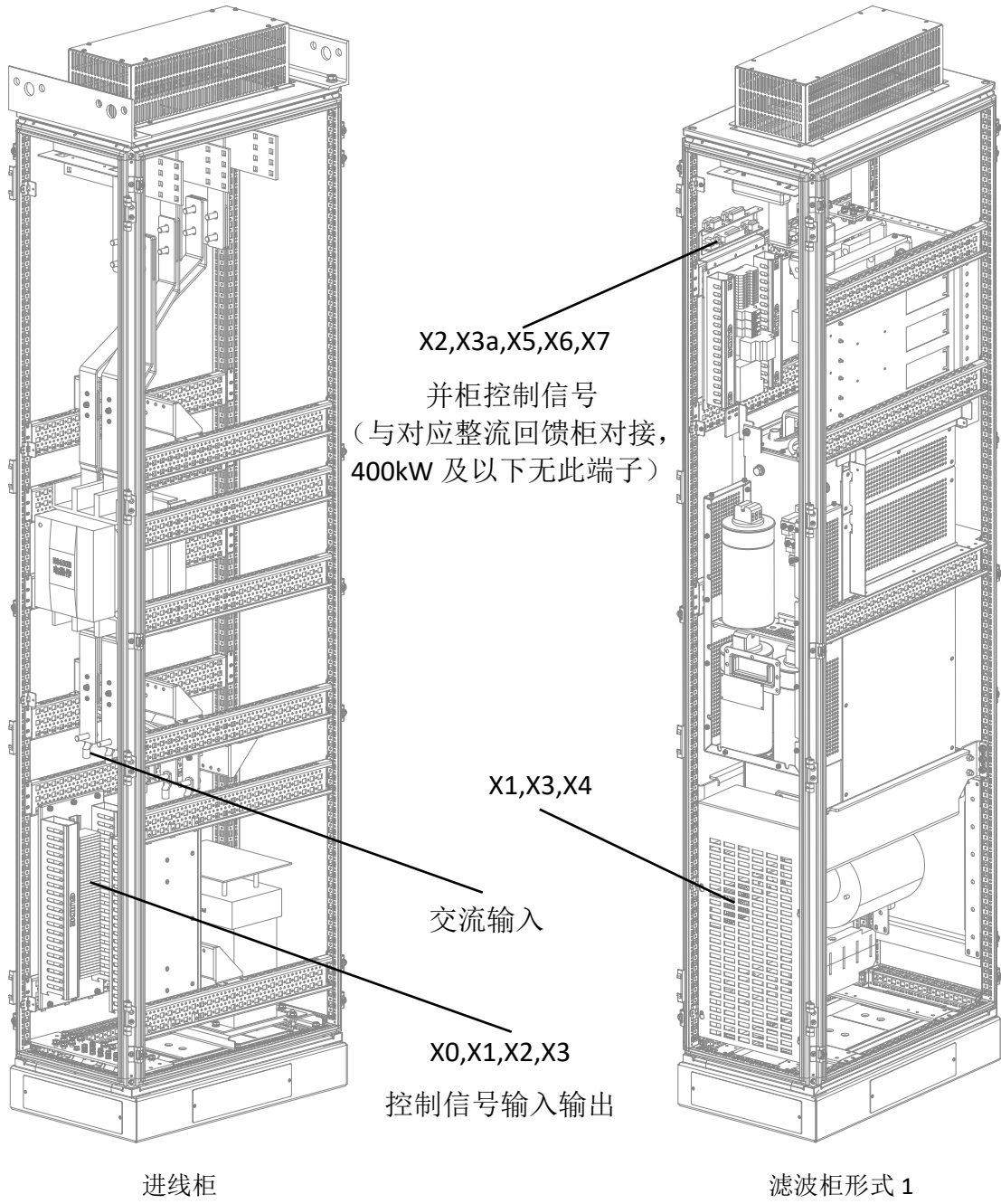
整流回馈标准成柜接线端子位置示意图 (a)
