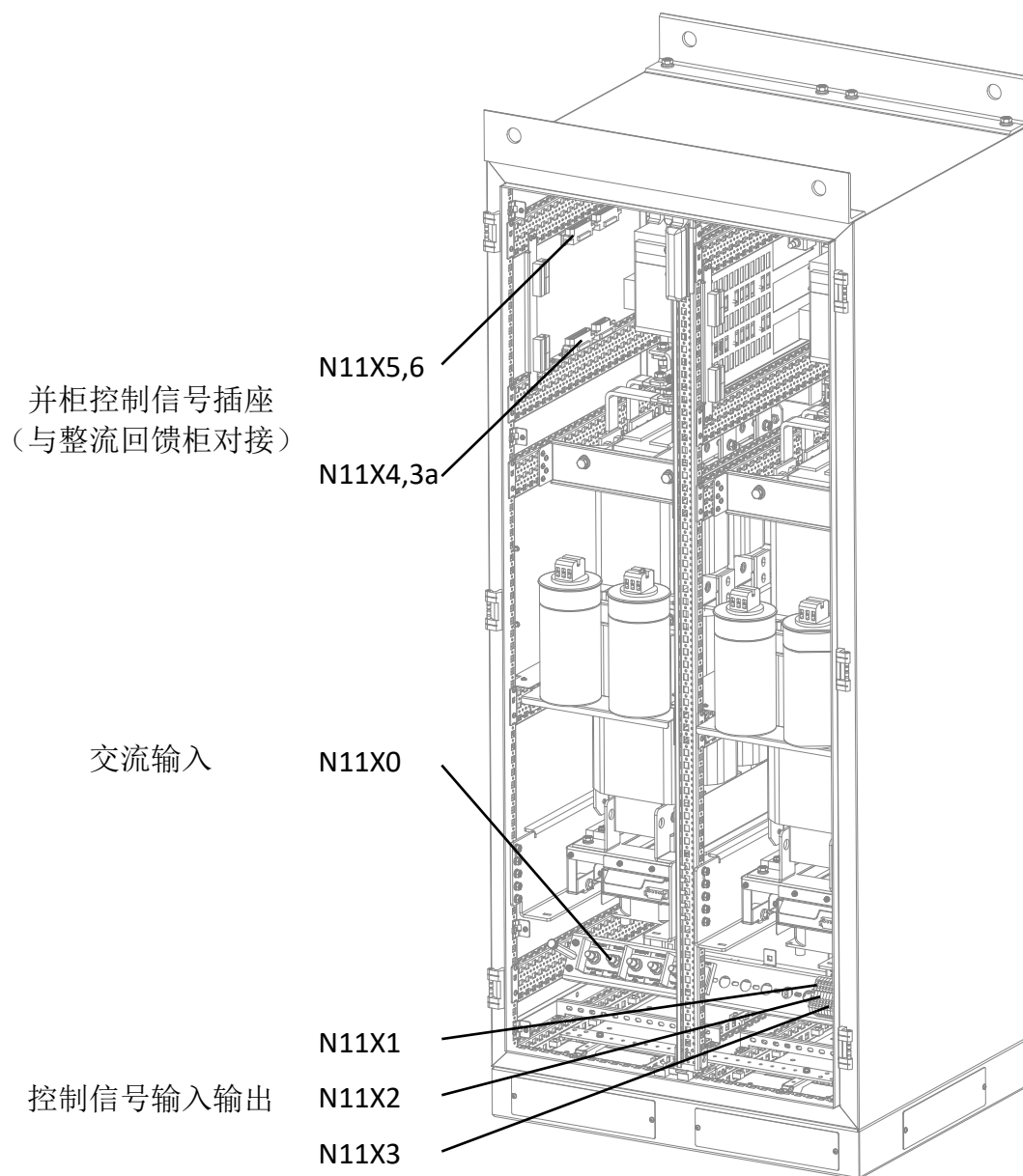
整流回馈 400kW 以上 C1、C4 成柜产品滤波柜接线端子位置示意图
