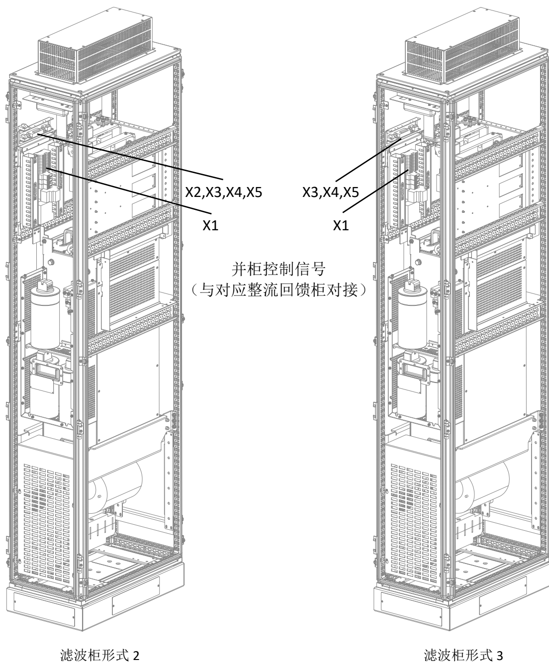
整流回馈标准成柜接线端子位置示意图 (b)
