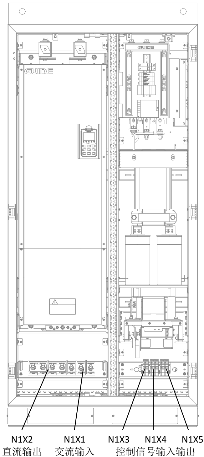
整流回馈 400kW 及以下 C1~C4 成柜产品接线端子位置示意图
