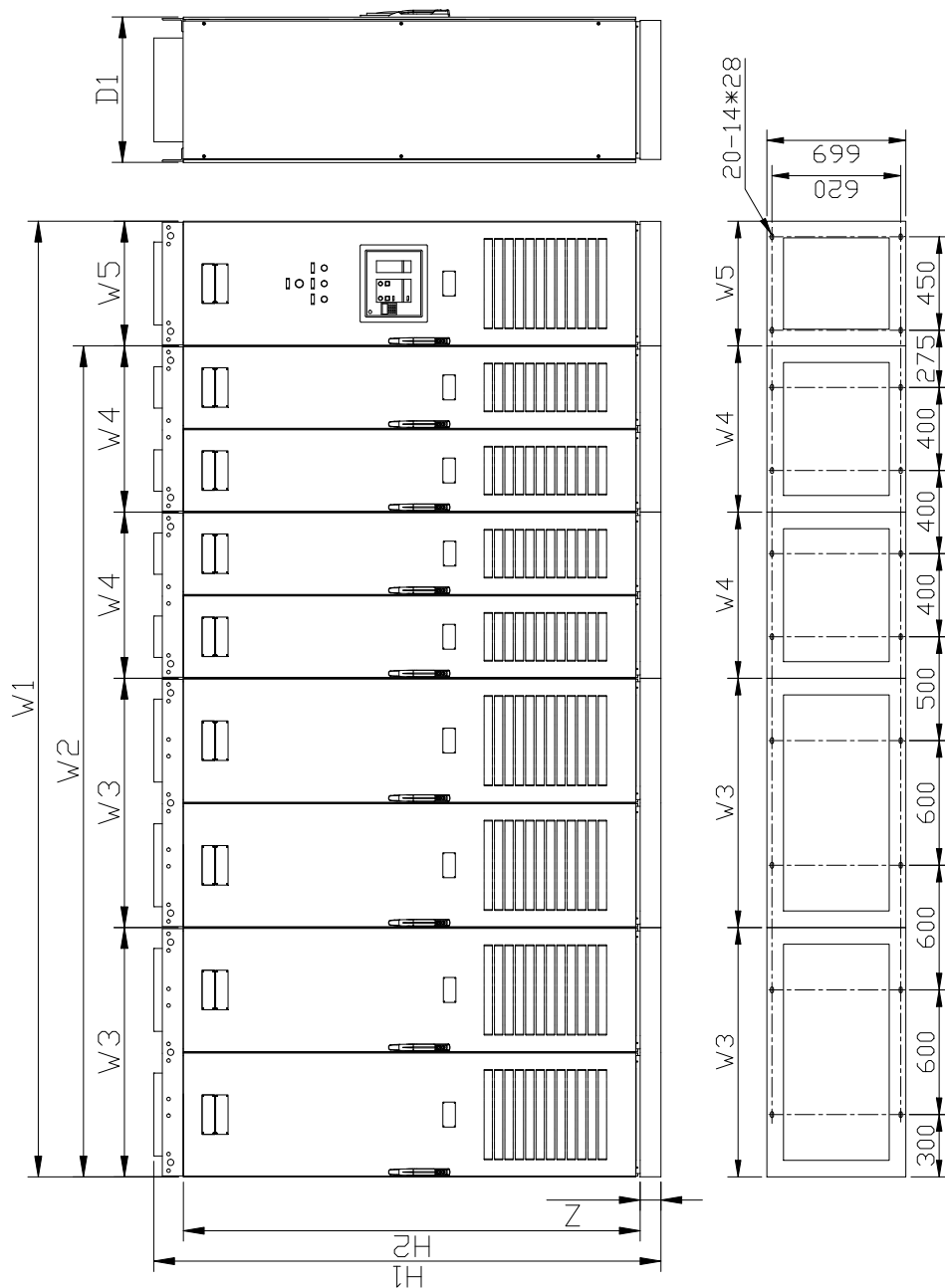
整流回馈 HF500A-1600-4-C 成柜外形示意图
