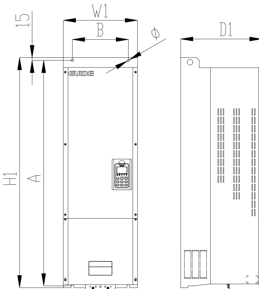
逆变器 HF500B-160-4-D、HF500B-185-4-D 和 HF500B-200-4-D 外形示意图
