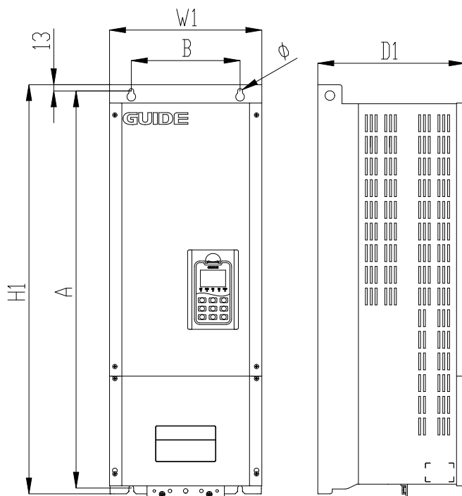
逆变器 HF500B-075-4-D 和 HF500B-090-4-D 外形示意图
