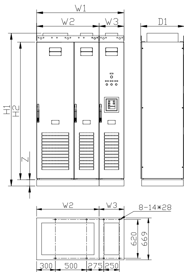
整流回馈 HF500A-250-4-C、HF500A-315-4-C 和 HF500A-400-4-C 成柜外形示意图
