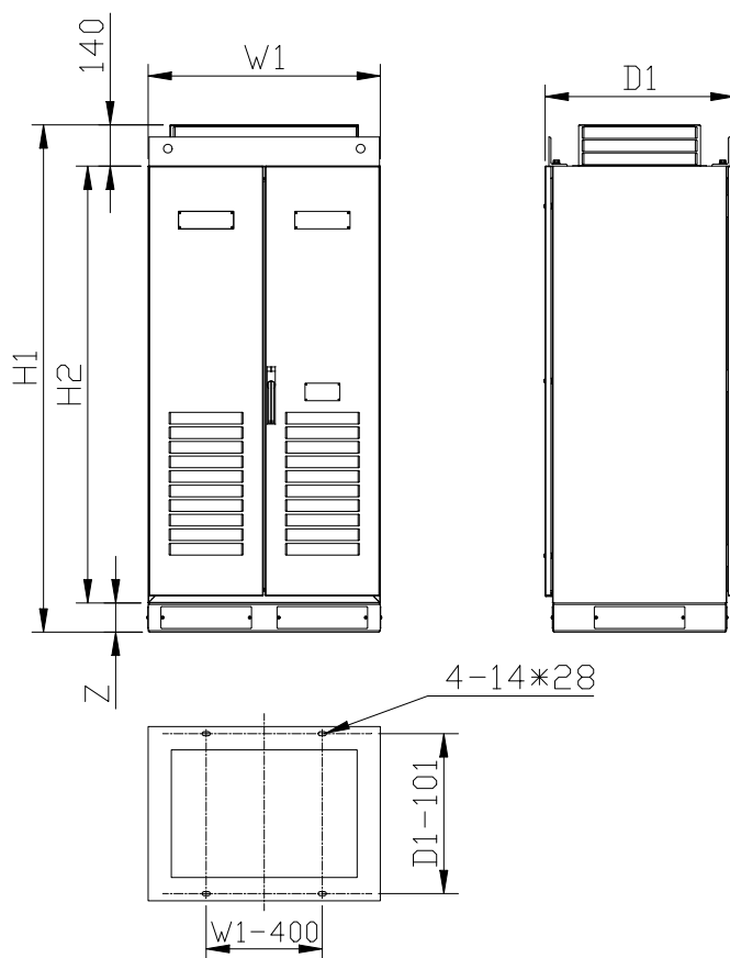
整流回馈 HF500A-075-4-C4、HF500A-132-4-C4、HF500A-250-4-C4、 HF500A-315-4-C4 和 HF500A-400-4-C4 成柜外形示意图
