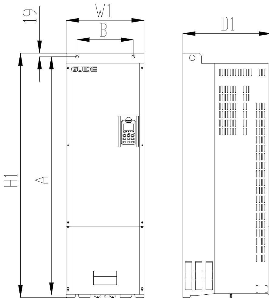
逆变器 HF500B-220-4-D 和 HF500B-250-4-D 外形示意图
