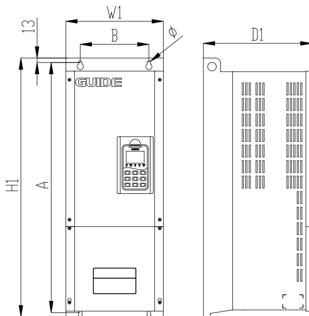
逆变器 HF500B-037-4-D、HF500B-045-4-D 和 HF500B-055-4-D 外形示意图
