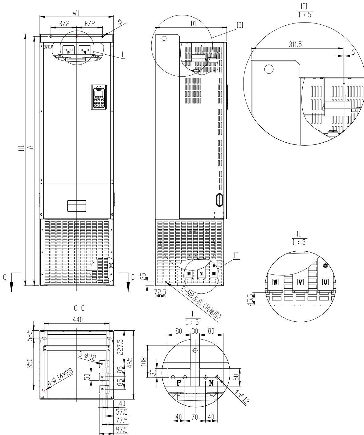
逆变器 HF500B-315-4-D、HF500B-355-4-D 和 HF500B-400-4-D 外形示意图
