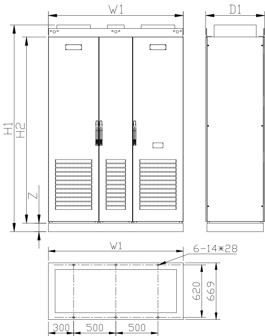
逆变器 HF500B-630-4-C、HF500B-800-4-C 外形示意图
