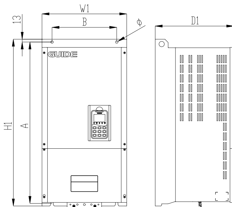
逆变器 HF500B-110-4-D 和 HF500B-132-4-D 外形示意图
