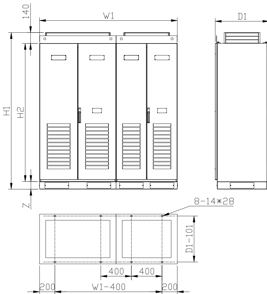
整流回馈 HF500A-500-4-C4、HF500A-630-4-C4 和 HF500A-800-4-C4 成柜外形示意 图
