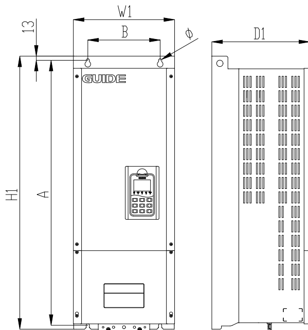
整流回馈 HF500A-075-4-D 外形示意图
