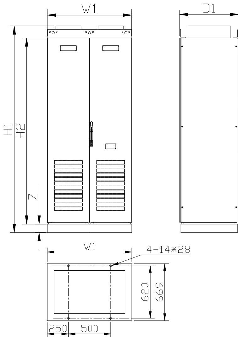
逆变器 HF500B-500-4-C 外形示意图
