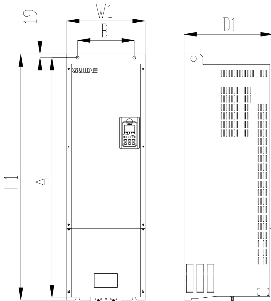
整流回馈 HF500A-250-4-D 外形示意图
