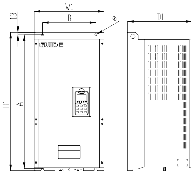
整流回馈 HF500A-132-4-D 外形示意图
